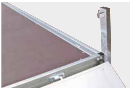
Rongzakken en afneembare hoekprofielen, beide in het dompelbad thermisch verzinkt
